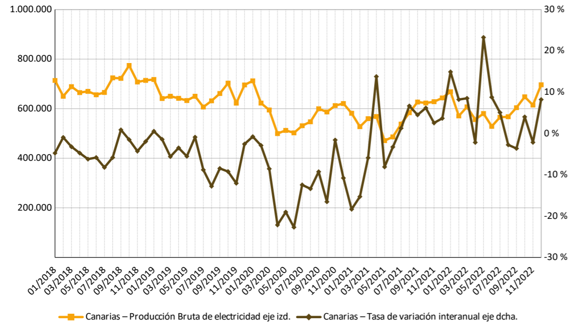
GRÁFICO 4.14. EVOLUCIÓN DE LA PRODUCCIÓN BRUTA DE ELECTRICIDAD EN CANARIAS. (Mwh y tasa de variación interanual). 2018-2022
