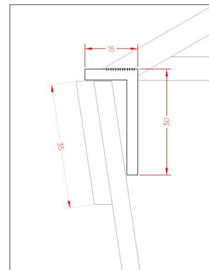
Detalle E 1:1
