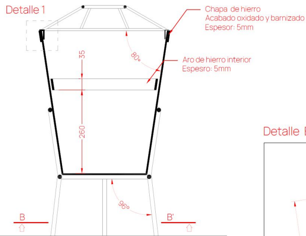
SECCIÓN A-A'
