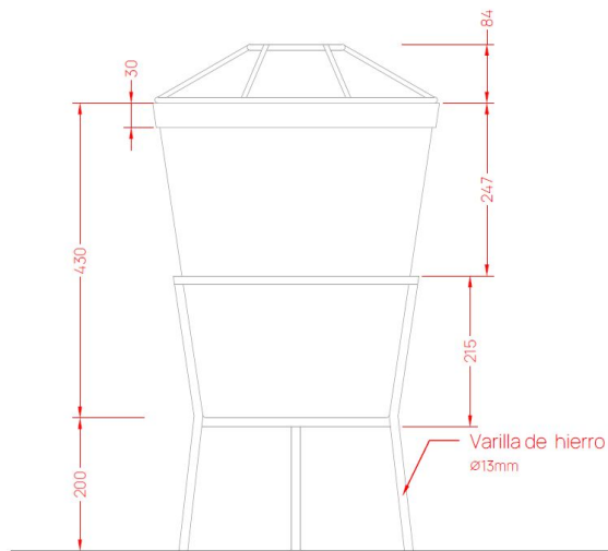
ALZADO
