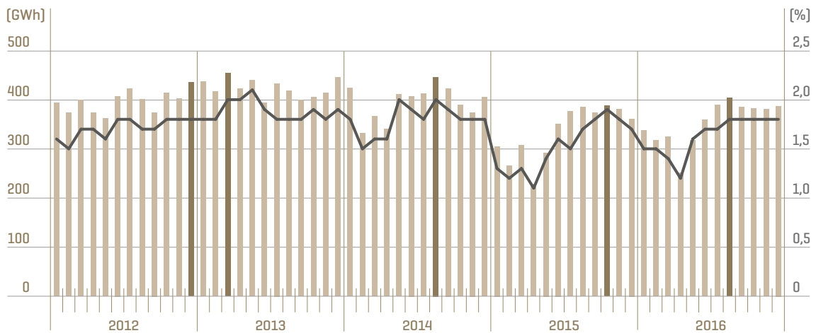
■ Generación resto de renovables [GWh] ■ Máximo mensual [GWh] — Generación resto de renovables / Generación total [%] [1] Incluye biogás, biomasa, geotérmica, hidráulica marina, hidroeléctrica y residuos renovables. // Fuente: REE. Datos de islas Baleares e islas Canarias disponibles desde 2006 y Ceuta y Melilla desde 2007.
