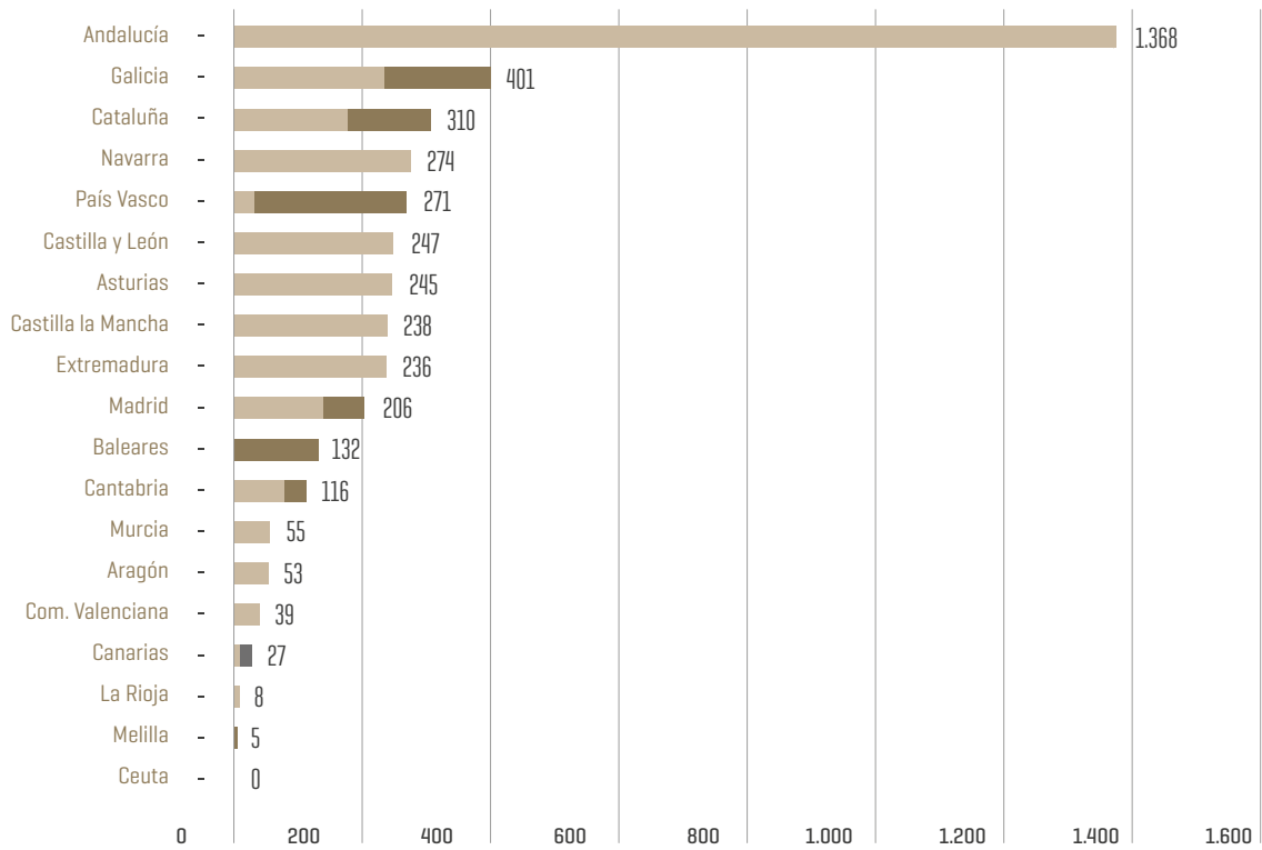
■ Otras renovables [1] ■ Residuos renovables ■ Hidroeléctrica [1] Incluye biogás, biomasa, geotérmica e hidráulica marina. // Fuente: REE.
