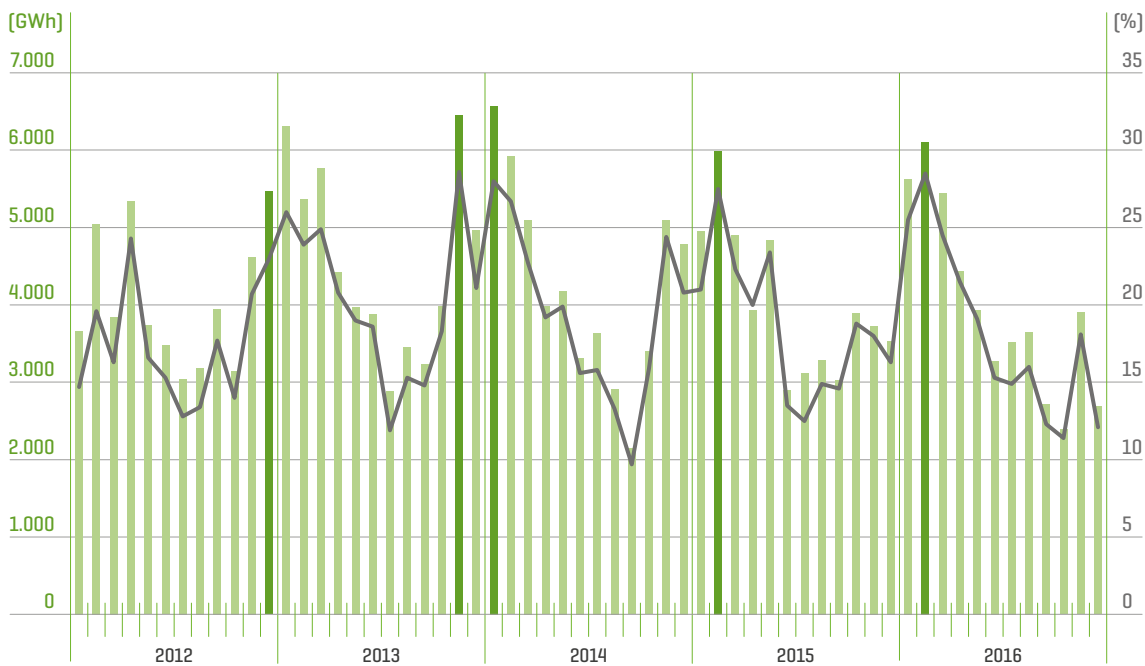
[GWh] [%] GENERACIÓN EÓLICA NACIONAL, MÁXIMOS MENSUALES Y PARTICIPACIÓN EN LA GENERACIÓN TOTAL SISTEMA ELÉCTRICO NACIONAL
